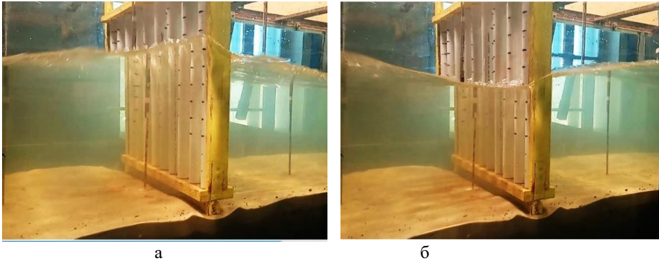
Рис. 4. Проходження гребня (а) та впадини (б) гравітаційної хвилі через проникну вертикальну стінку проникністю 50%
