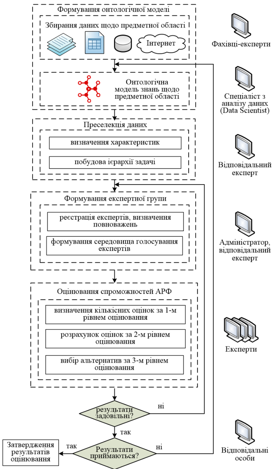
Рис. 3 – Алгоритм проведення оцінювання спроможностей АРФ
